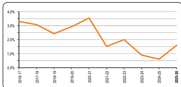
kVA dañados vs instalados en SET rurales
